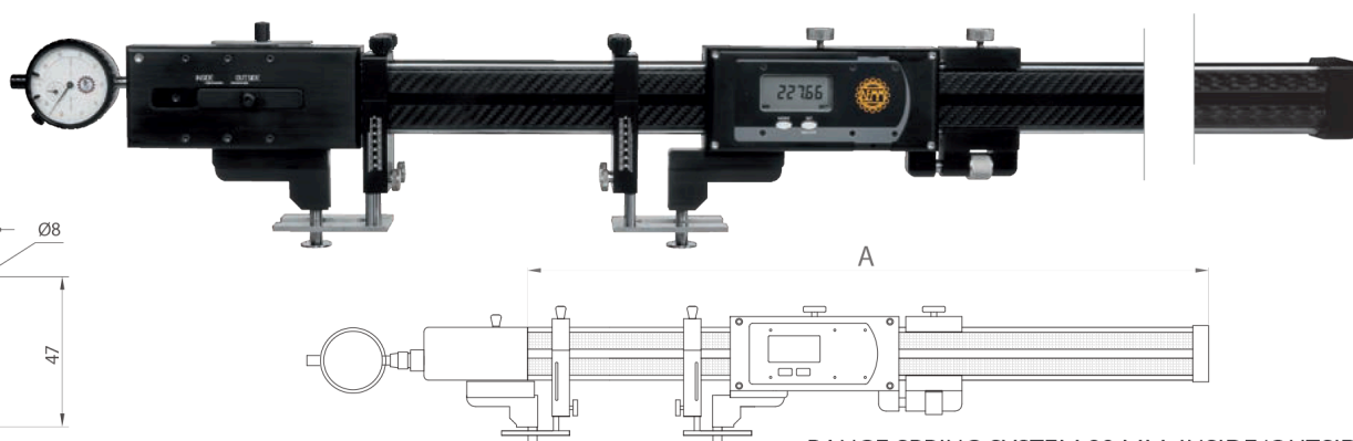
CARBON BAR SECTION SEZIONE ASTA IN CARBONIO
