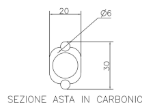
SEZIONE ASTA IN CARBONIO
