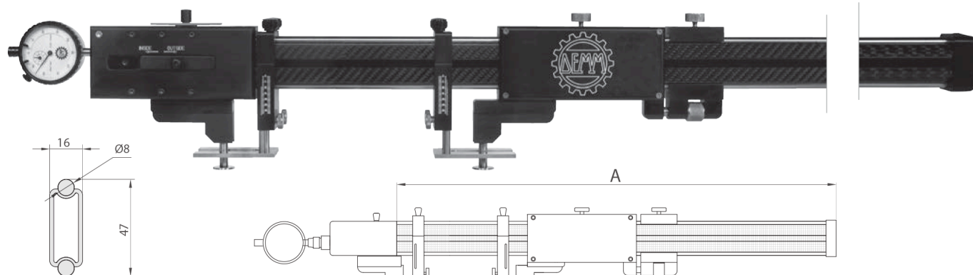
CARBON BAR SECTION SEZIONE ASTA IN CARBONIO
